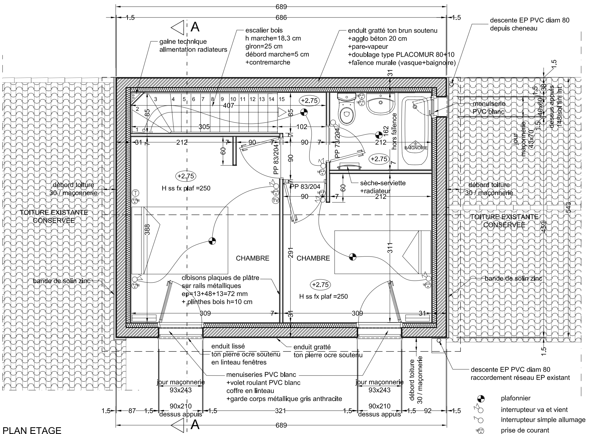
PLAN ETAGE
